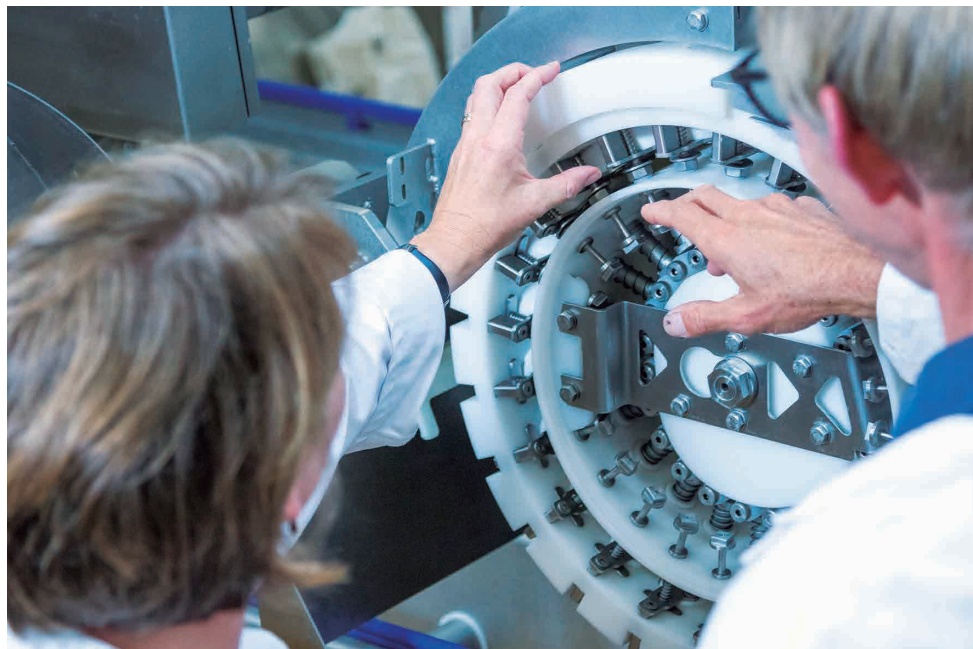
Roda de Extrusão - Extrusion-wheel
